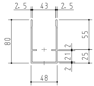
アルミチャンネル 40-80-25H
