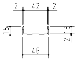
アルミチャンネル 40-15H
