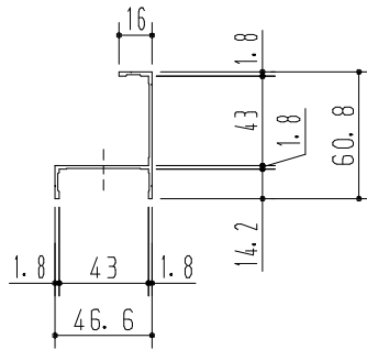
アルミチャンネル 40-F
